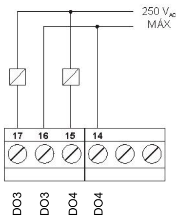
Figura 14 - Ligação das saídas digitais.
