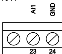
Figura 9 - Conexão da entrada analógica.
