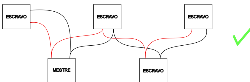
Figura 4 - Ligação encadeada ( Daisy Chain ).
