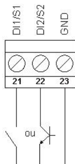
Figura 10 - Uso das entradas digitais.
