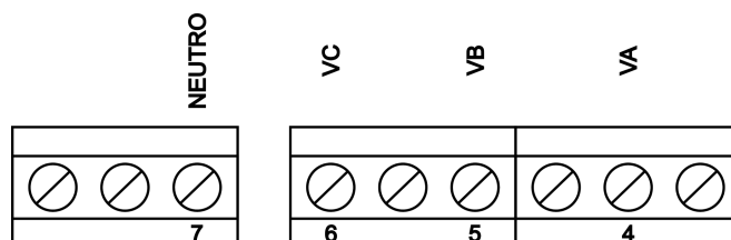
Figura 6 - Conexões para medição de tensão.
