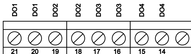
Figura 12 - Conexão das saídas digitais.
