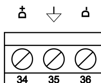
Figura 3 - Conexão da comunicação RS485.
