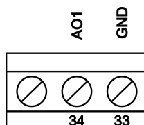
Figura 13 - Conexão da saída analógica.
