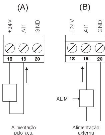
Figura 11 - Ligação da entrada analógica.
