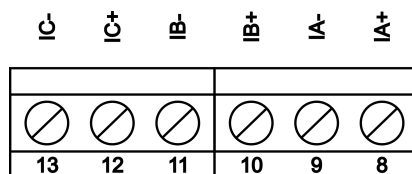
Figura 7 - Conexões para a medição de corrente.
