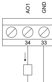
Figura 15 - Conexão da saída analógica.
