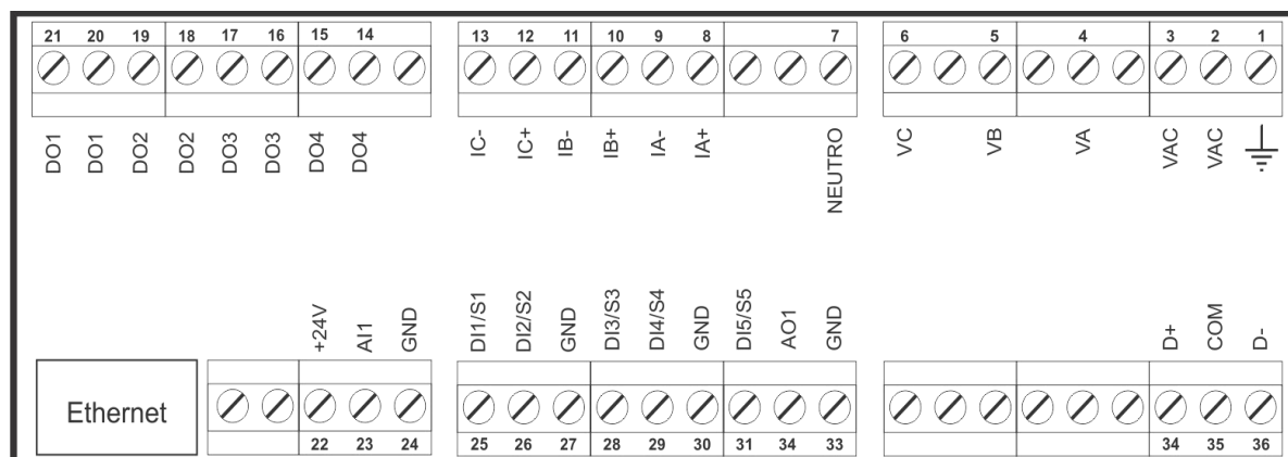
Figura 1 - Conexões do produto.
