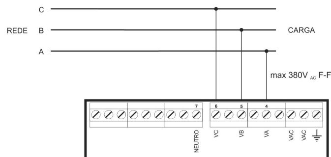
Figura 14 - Diagrama de ligações.
