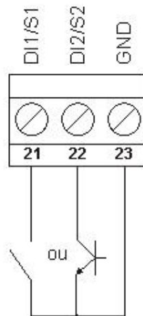
Figura 9 - Uso das entradas digitais.
