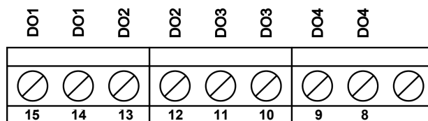
Figura 11 - Conexão das saídas digitais.
