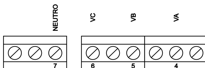
Figura 6 - Conexões para medição de tensão.
