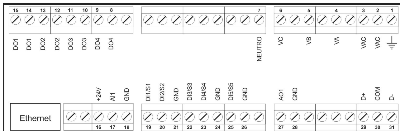
Figura 1 - Conexões do produto.
