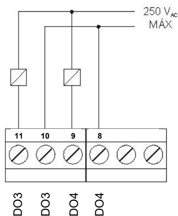
Figura 13 - Ligação das saídas digitais.
