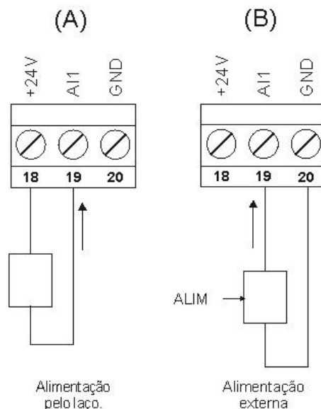
Figura 10 - Ligação da entrada analógica.
