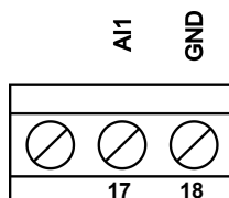
Figura 8 - Conexão da entrada analógica.
