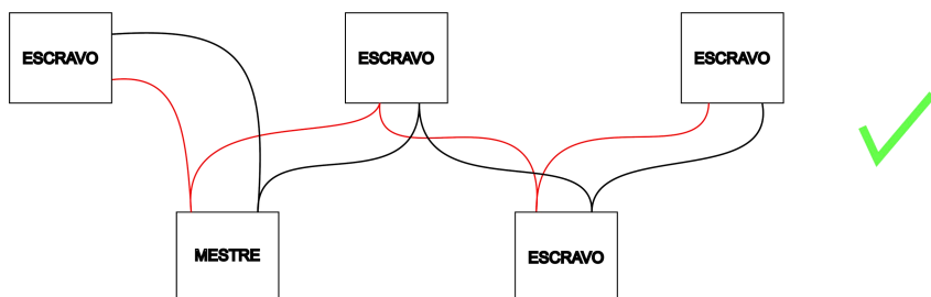
Figura 13 - Ligação encadeada ( Daisy Chain ).
