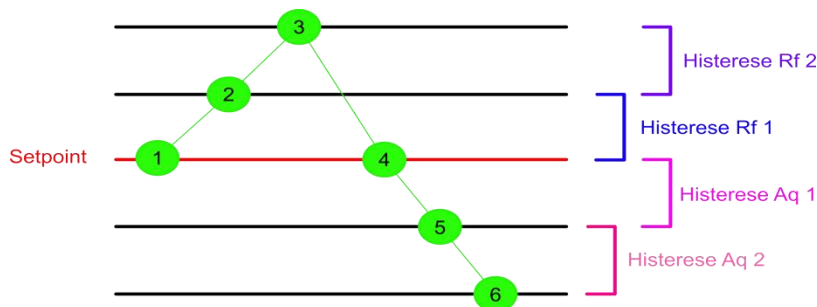
Figura 233 - Funcionamento dos estágios de refrigeração e aquecimento.
