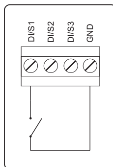
Ligação de contato seco
