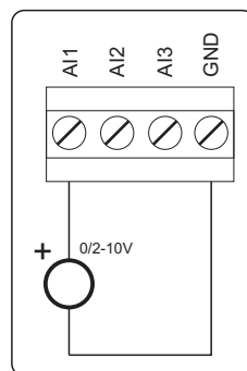
Ligação de sensor com saída em tensão
