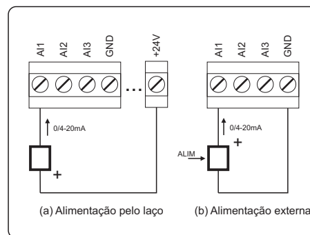
Ligação de sensor com saída em corrente
