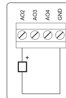
Saídas analógicas (tensão ou corrente)
