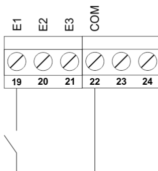
Figura 5 - Uso das entrada universais para contato seco.
