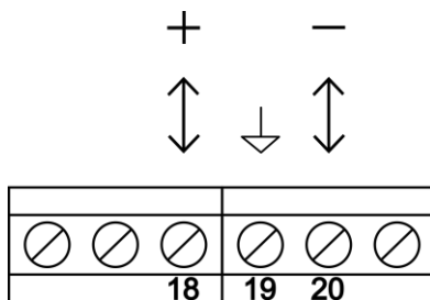
Figura 13 - Conexão da comunicação RS485 principal.
