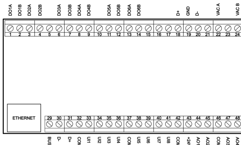
Figura 2 - Conexões do MCP18-ETH.
