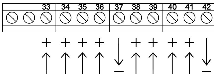
Figura 4 - Conexão das entradas universais.
