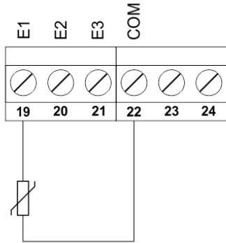
Figura 6 - Uso das entradas universais para sensores NTC.
