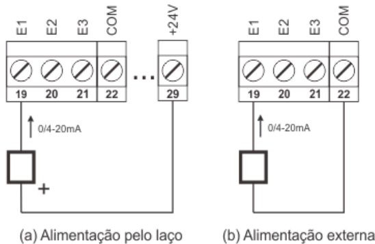
Figura 7 - Uso das entradas universais para sinais de corrente.
