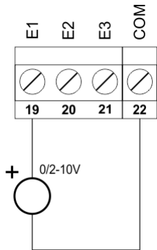
Figura 8 - Uso das entradas universais para sinais de tensão.
