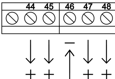
Figura 10 - Conexão das saídas analógicas.
