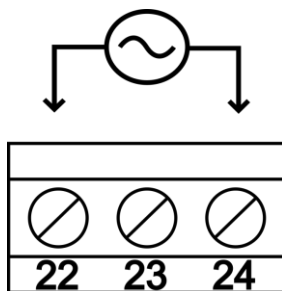
Figura 3 - Conexão da alimentação.
